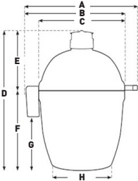
SEITENANSICHT
